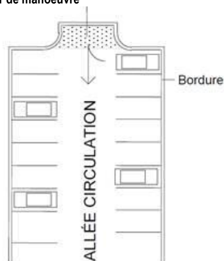
Figure 6.1 : Surlargeur de manoeuvre
